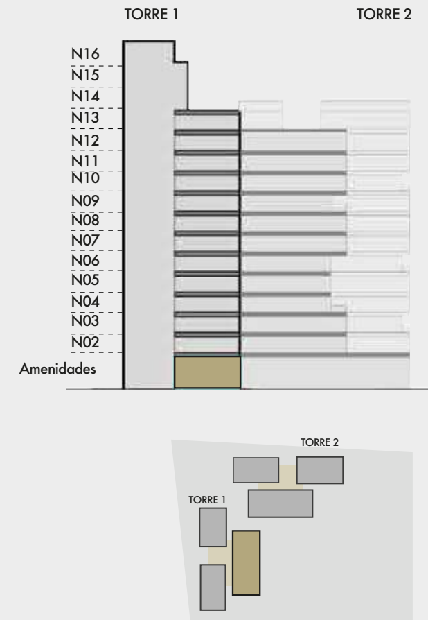
PLANTA ALTA
